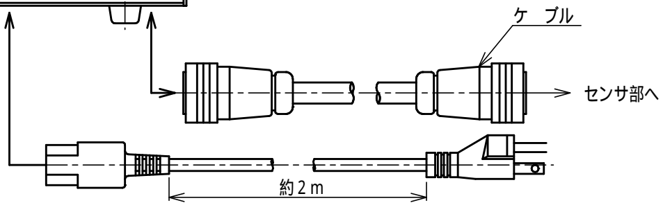
露点計 DPH-503B型 表示部
