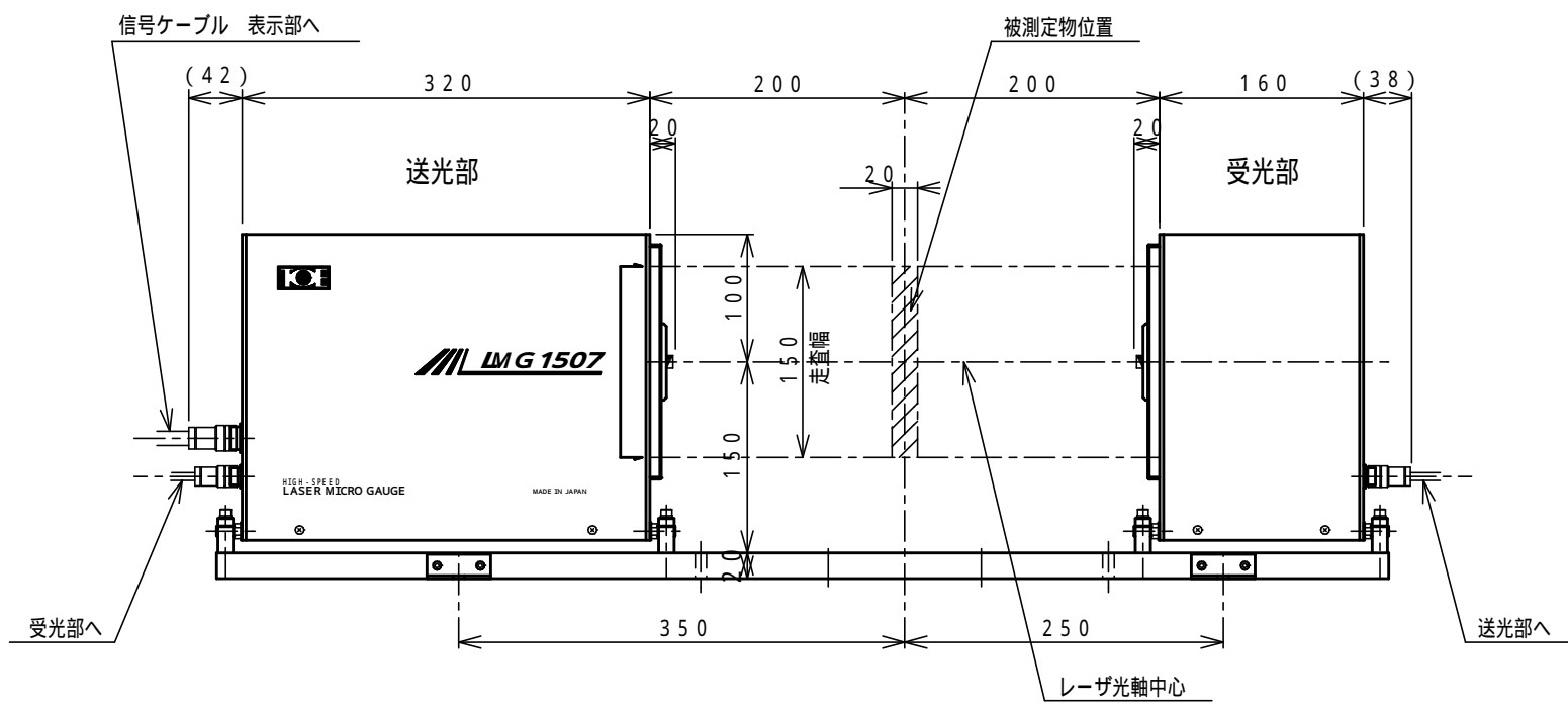
LMG 1507 センサ部
