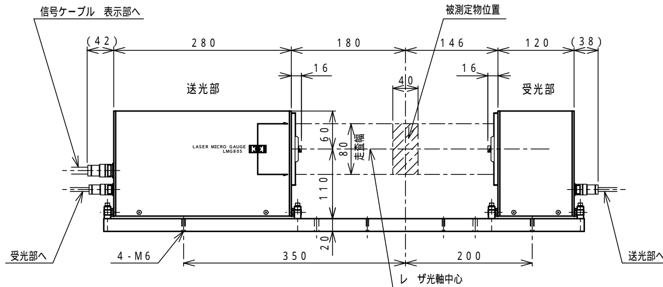
LMG805 センサ部
