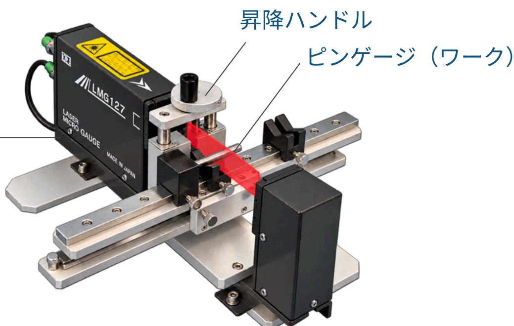
外径寸法 測定器 LMG-127
