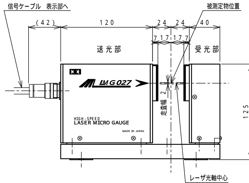
LMG027 センサ部
